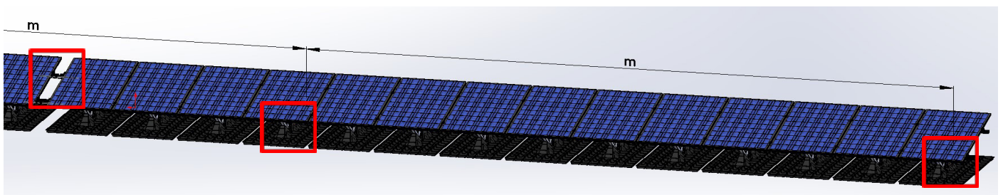
Anwendungsbeispiel Blitzschutz auf Contec.greenlight
